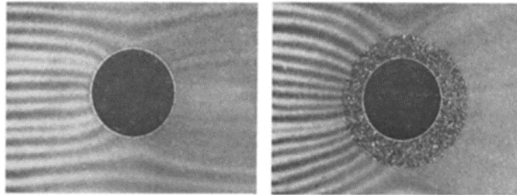
Figure 26 : Illustration de l'effet d'un forage sur l'écoulement en milieu poreux (Drost et al. 1968).
