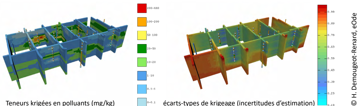
Résultat de traitement : krigeage 3D de teneurs en polluant et incertitude associée.
